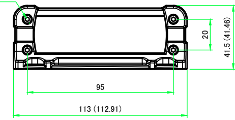
A-A (1:2.5)
