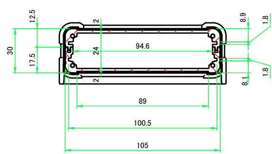
A-A (1:2.5)
